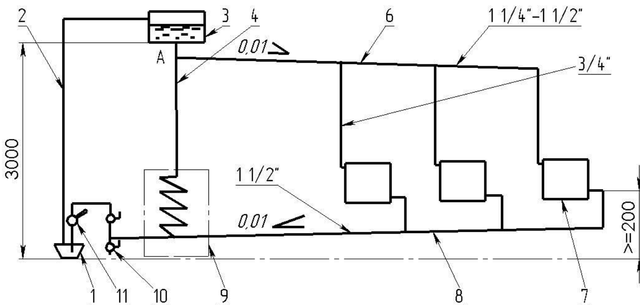
Рис. 2 Схема водяной системы с естественной циркуляцией воды.
